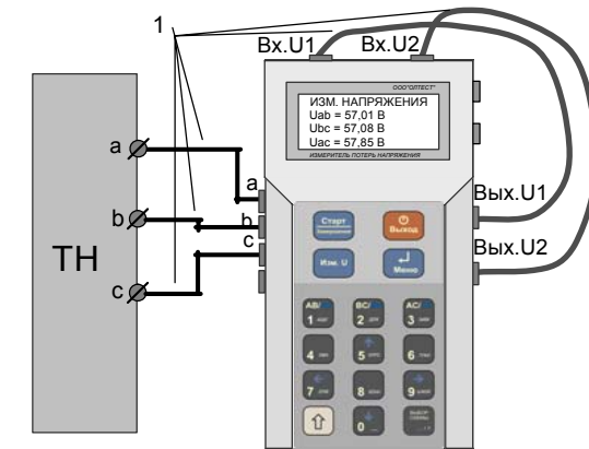
Рисунок 6.2. Варианты подключения стационарного блока к ТН
