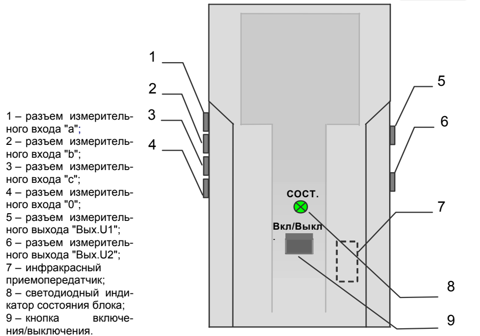
Рисунок 5.2. Вид стационарного блока Измерителя
