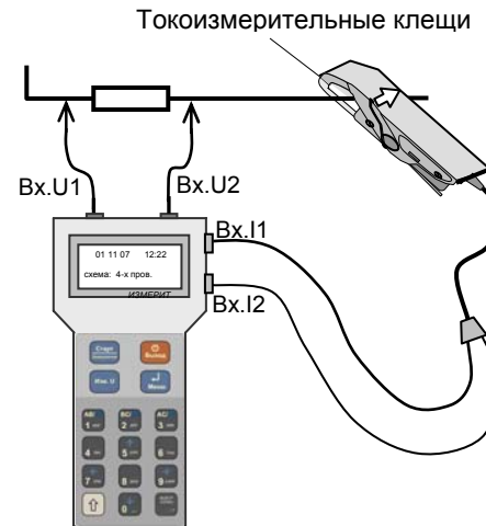
Рисунок 6.5. Подключение переносного блока Измерителя при измерении силы тока
